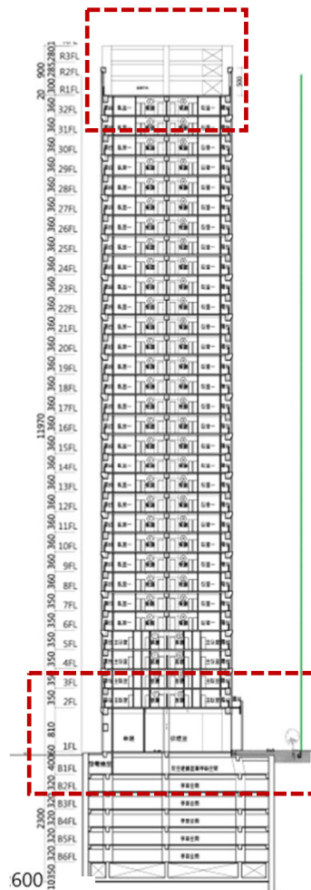
圖9-23 全區剖面圖
