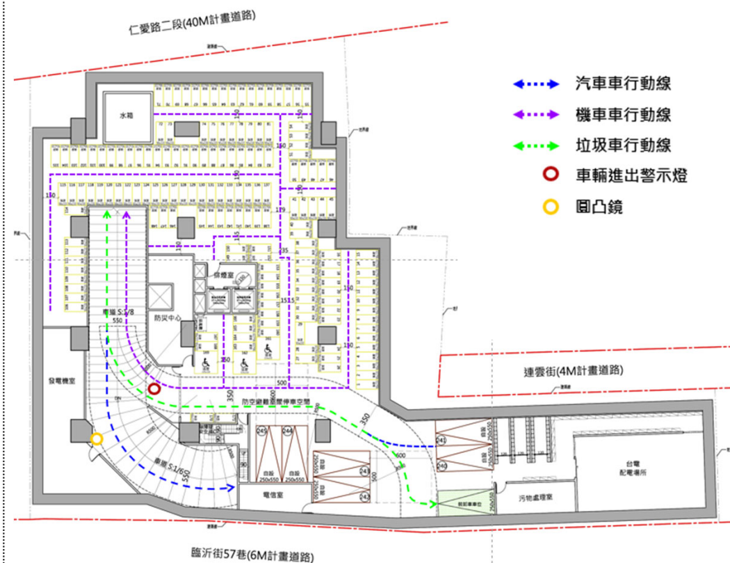
圖9-15 地下一層平面圖
